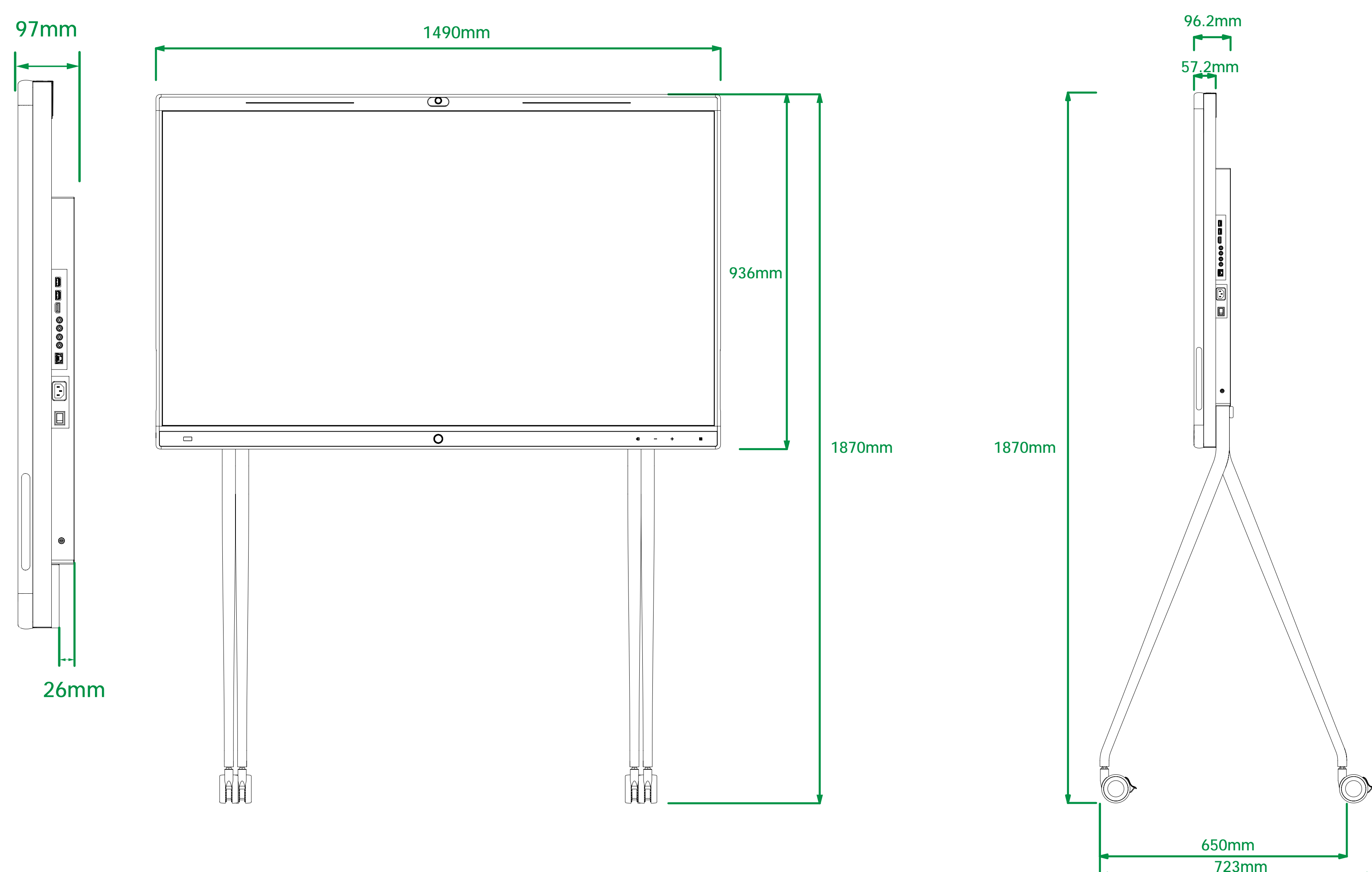
Dimensions du pied à roulette
